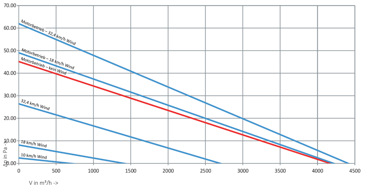
Geprüfte Kennlinien
